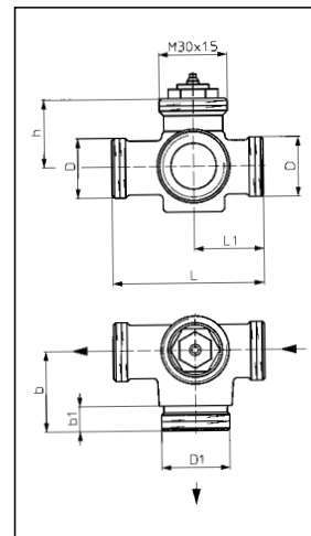
правостороннее присоединение
