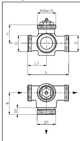
левостороннее присоединение
