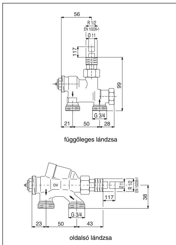
Lánczásszelep (egycsöves/kétcsöves)
