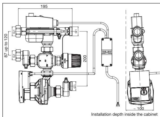
Dimensions
