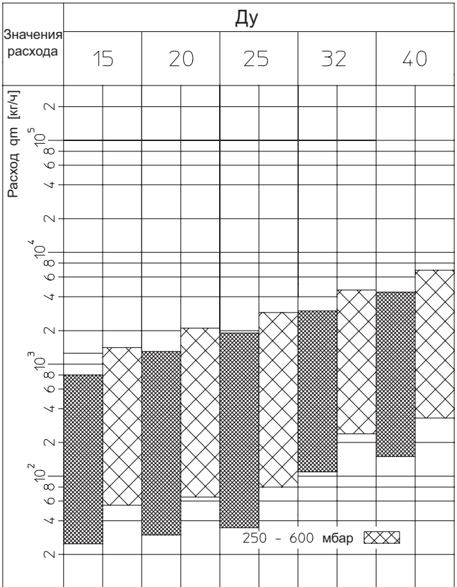
Значения расхода на регуляторе перепада давления „Нусосон DP“ при перепаде давления в стояке от 50 до 300 мбар или от 250 до 600 мбар с дополнительным ограничением расхода на регулирующем вентиле „Нусосон V“.
