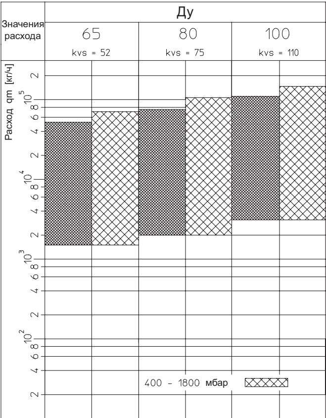
Значения расхода на регуляторе перепада давления „Нусосон DP“ при перепаде давления в стояке от 200 до 1000 мбар или от 400 до 1800 мбар.
