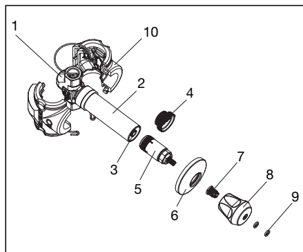
Fig. 6.1 Robinet pour pose encastrée avec fourreau à encastrier
