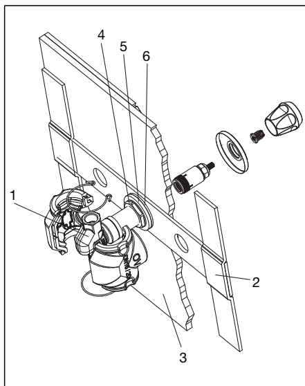
Abb. 6.5 Rückseite Trockenbauinstallation
