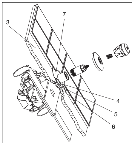
Abb. 6.6 Vorderseite Trockenbauinstallation
