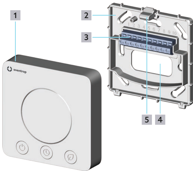
Abb. 3: Aufbau F 210, F 310
