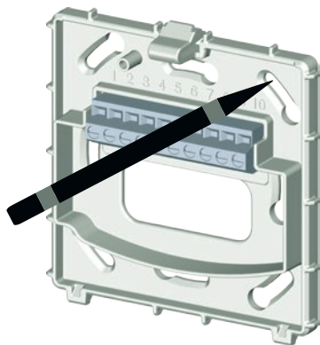
Abb. 8: Montageplatte montieren
