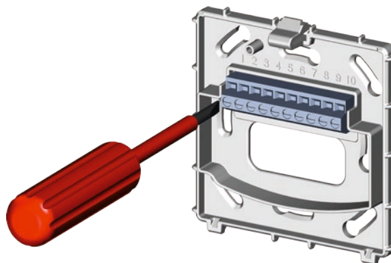
Abb. 9: ClimaCon F elektrisch anschließen
