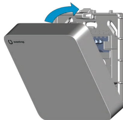
Abb. 10: Bedieneinheit aufsetzen
