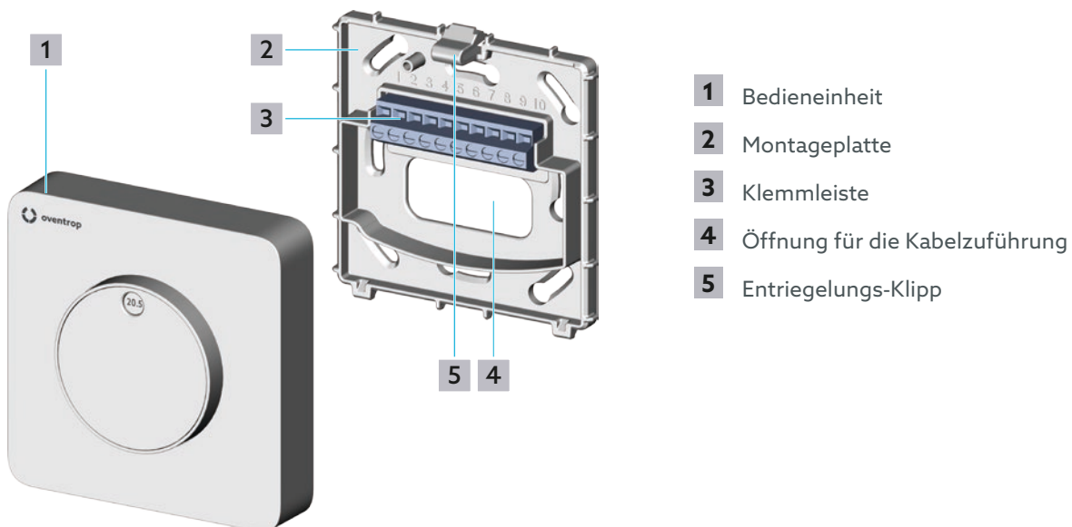
Abb. 2: Aufbau F 90, F 100
