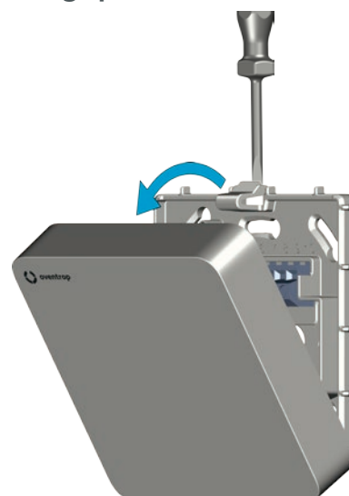
Abb. 7: Montageplatte lösen
