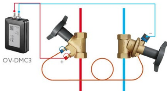
Bild 7: Kopplingsschema OV-DMC3
