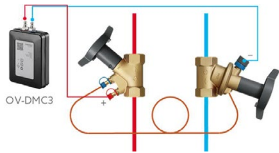
Afb. 7: Aansluitschema OV-DMC3
