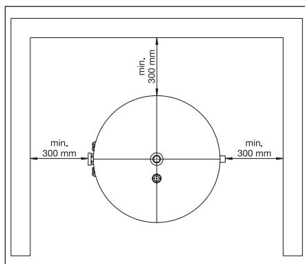
Fig. 5.1 Ecartements minimaux vers le mur
