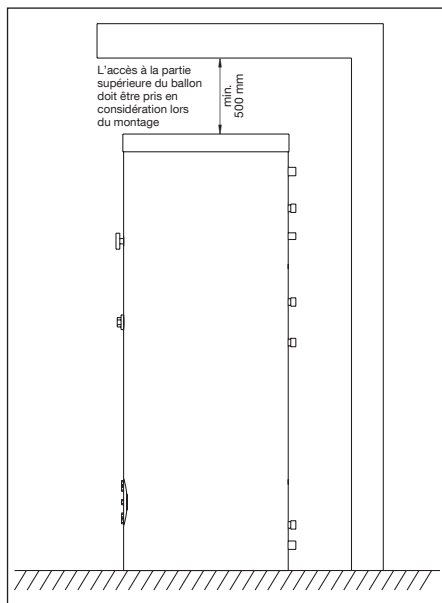
Fig. 5.2 Ecartement minimal vers le plafond
