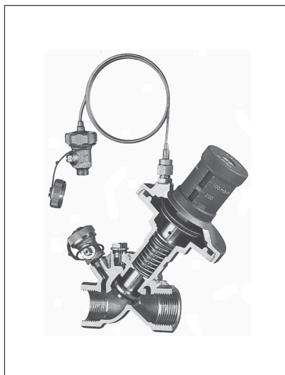
Schematische doorsnede
