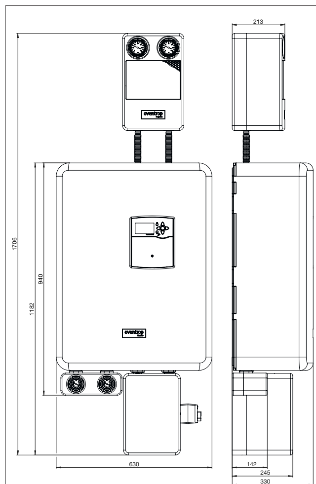
Fig. 3: Encombres en mm
