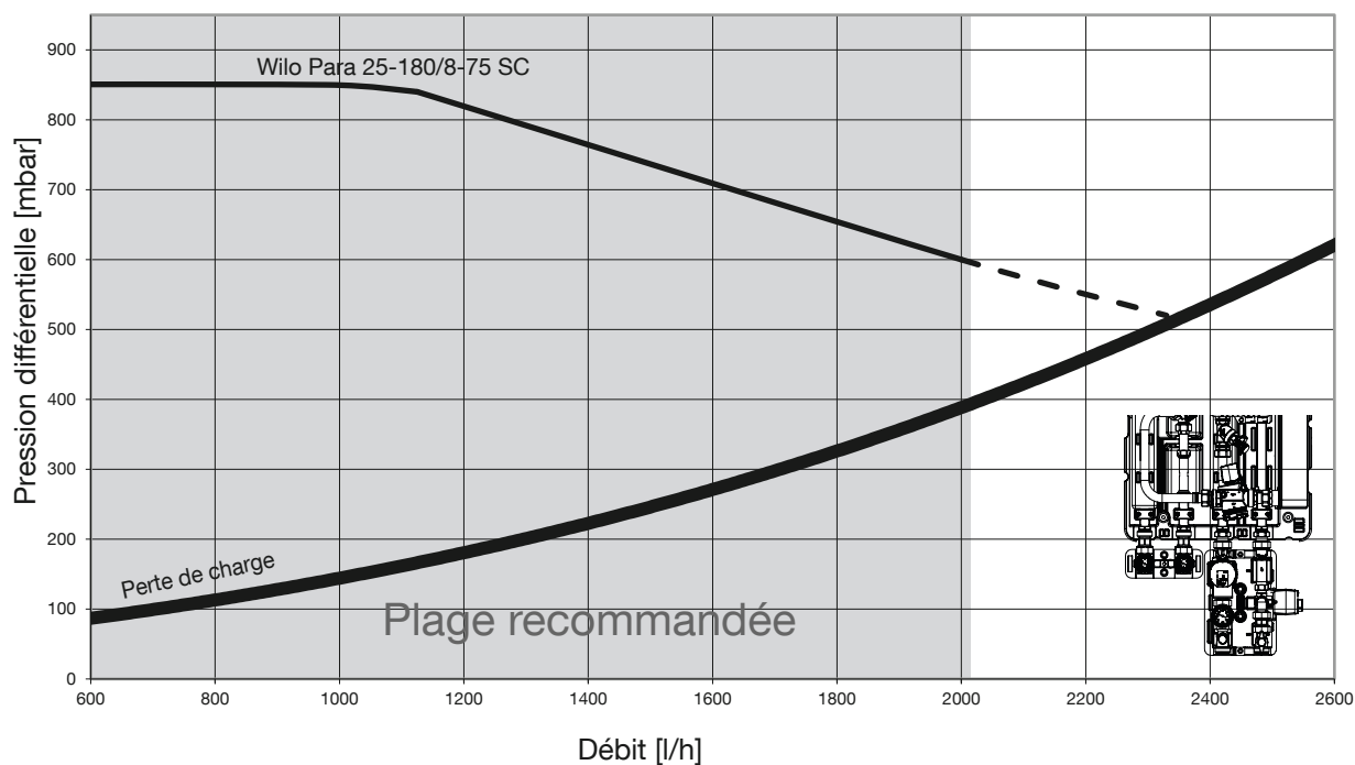
Fig. 6: Perte de charge circuit secondaire Regudis H-MHT (module de commutation HT)
