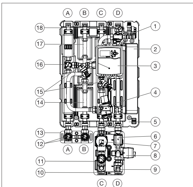
Fig. 2: Configuration Regudis H-MT
