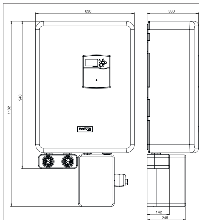
Fig. 3: Encombres en mm
