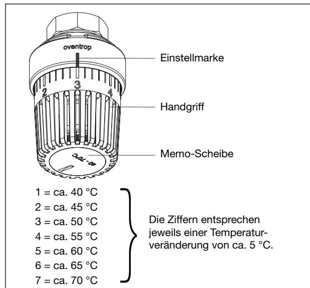
Temperaturregler
