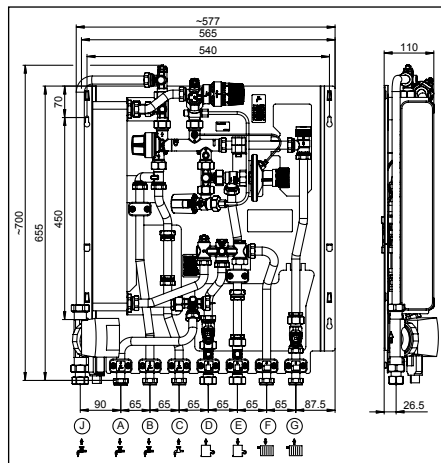
Fig. 4.2 Encombresments avec circuit de chauffage direct et conduite de bouclage d'E.C.S.
