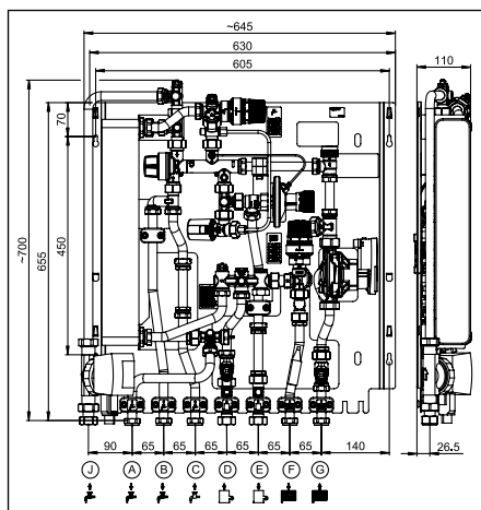
Fig. 4.3 Encombresments avec circuit de chauffage mélangé et conduite de bouclage d'E.C.S.
