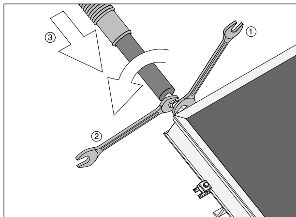
Fig. 2 Lors du serrage, maintenir le flexible de raccordement du capteur à l'aide d'une seconde clé pour éviter de détériorer le flexible ou le raccord du capteur. Enfiler le soufflet de protection sur l'isolation.
