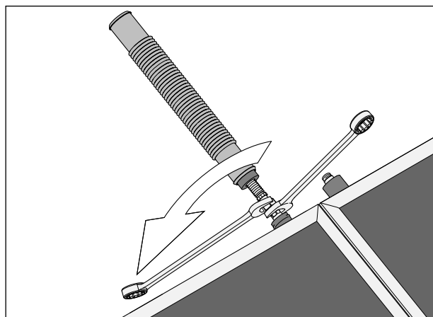
Fig. 4 Serrer le raccord d'1/4 de tour. Maintenir au serrage le raccord du capteur avec une seconde clé pour éviter de détériorer le raccord du capteur ou le flexible de liaison.
