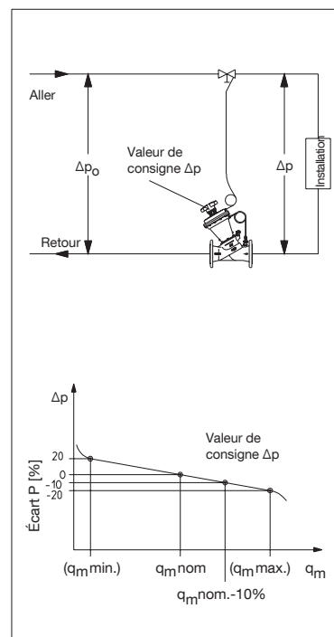
Schéma d'installation
