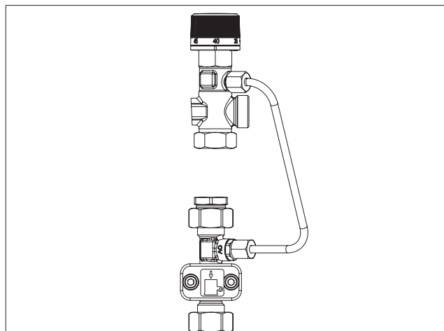
Abb. 5: Einbau Kupferrohr Regudis W-HTU/TU und Regudis W-HTF
