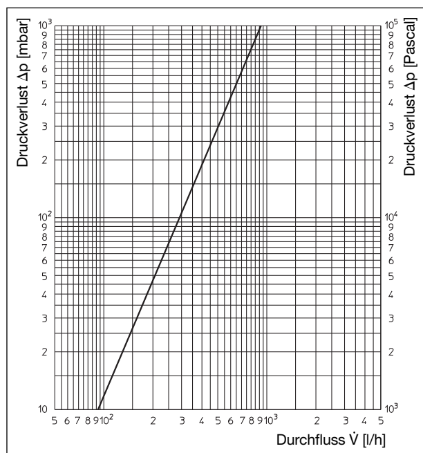
Durchflussdiagramm
