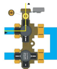
Vidange, purge et rinçage du côté installation
