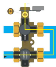
Remplissage et rinçage du côté appareil
