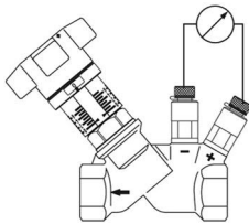
Mesure de la pression différentielle via le robinet HydroControl MTR. Permet de mesurer le débit sur la base de la pression différentielle via l'orifice de mesure HydroControl MTR et de la valeur kv enregistrée dans l'ordinateur de mesure OV-DMC 3.
