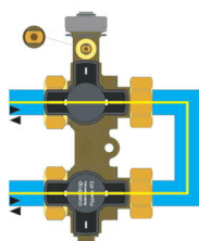
Fonctionnement normal
