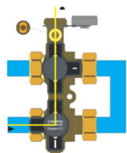
Vidange et purge du côté installation et du côtés appareil, rinçage du côté installation
