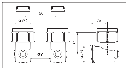
Fig. 6 Modèle équerre, G ¾ écrou x G ¾ mâle
