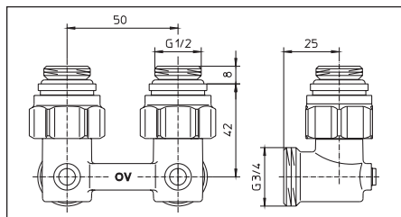
Fig. 7 Modèle équerre, G ½ mâle x G ¾ mâle
