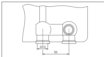
Fig. 8 Robinetterie intégrée G ½ femelle
