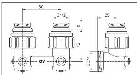
Abb. 7 Eckform, G \frac{1}{2} AG x G \frac{3}{4} AG
