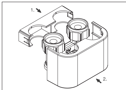
Abb. 10 Montage Design-Abdeckung
