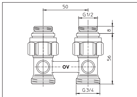
Fig. 5 Modèle droit, G ½ mâle x G ¾ mâle
