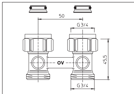
Fig. 4 Modèle droit, G ¾ écrou x G ¾ mâle
