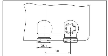
Abb. 9 Ventilgarnitur G \frac{3}{4} AG nach DIN EN 16313 (Eurokonus)
