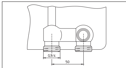
Fig. 9 Robinetterie intégrée G ¾ mâle selon DIN EN 16313 («eurocône»)
