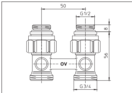
Abb. 5 Durchgangsform, G \frac{1}{2} AG x G \frac{3}{4} AG
