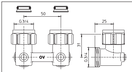
Abb. 6 Eckform, G \frac{3}{4} ÜM x G \frac{3}{4} AG
