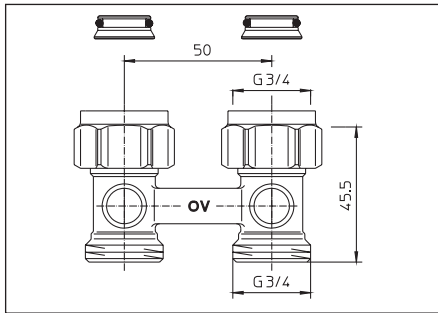
Abb. 4 Durchgangsform, G \frac{3}{4} ÜM x G \frac{3}{4} AG
