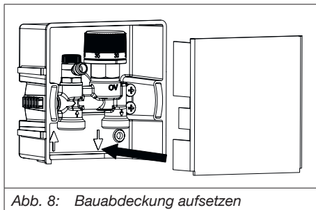
Abb. 8: Bauabdeckung aufsetzen
