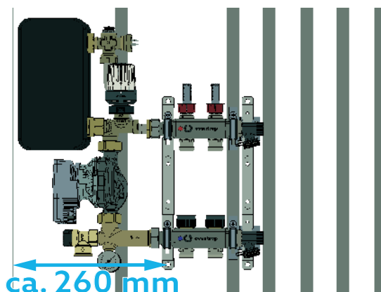
Abb. 9: Abstand Wand Einbauschränk und Heizkreisverteiler
