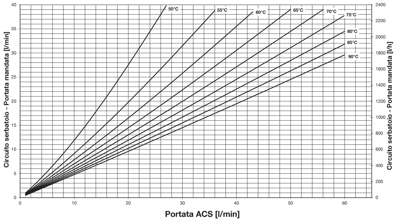
Fig. 41 - Portata in volume del circuito d'accumulo - Riscaldamento dell'acqua potabile a 50 °C
