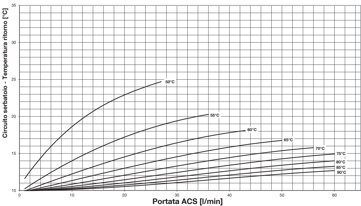
Fig. 42 - Temperatura di ritorno circuito d'accumulo - Riscaldamento dell'acqua potabile a 50 °C
