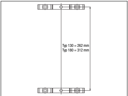
Abb. 6.6 Wandhalterungen befestigen
