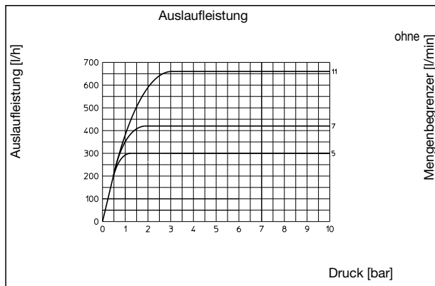
Durchflusskennlinie
