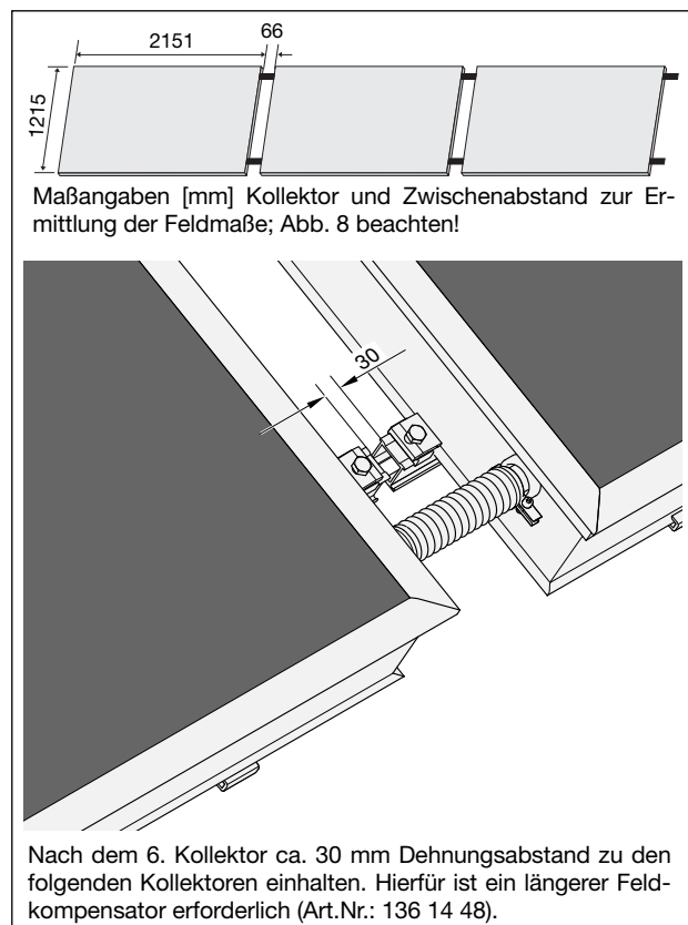
Abb. 8: Kollektorabstände
