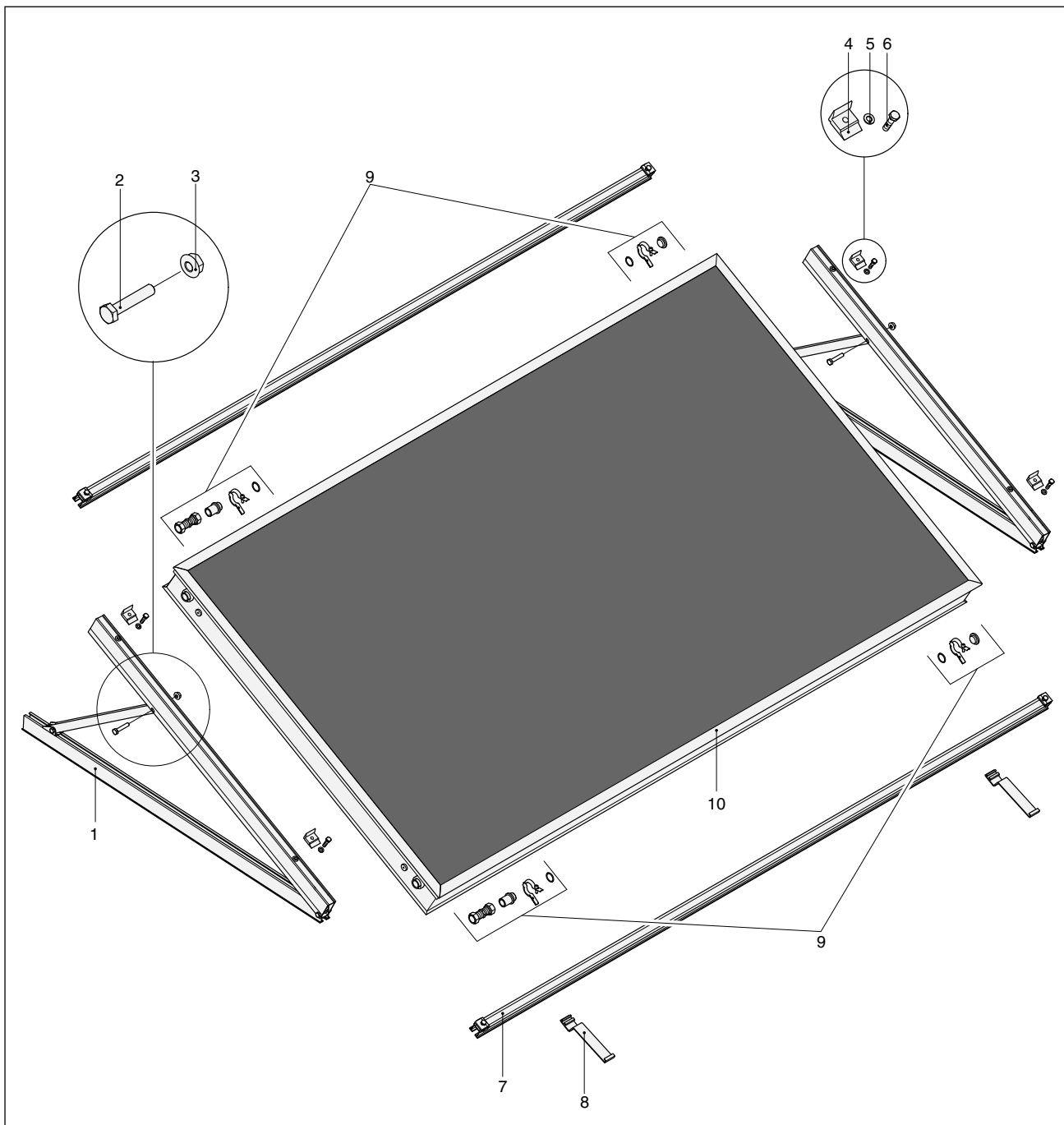
Abb. 19: Grundset Freiaufstellung
