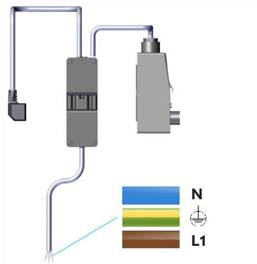
Abb. 7: Adernbelegung
