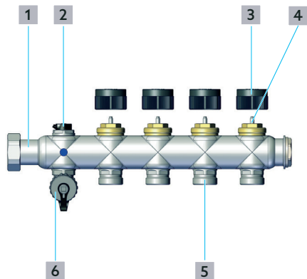
Fig. 2: Aufbau Rücklaufbalken
