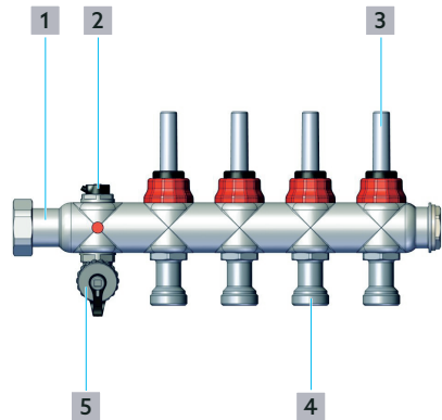
Fig. 1: Aufbau Vorlaufbalken
