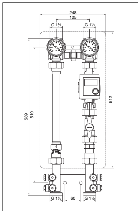
Fig. 4.2 Encombrements groupe de raccordement circuit de chauffage
