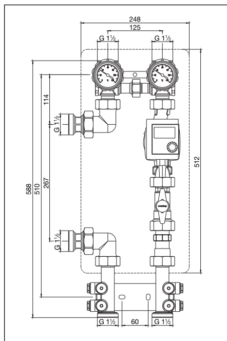
Fig. 4.1 Encombrements groupe de raccordement ballon tampon
