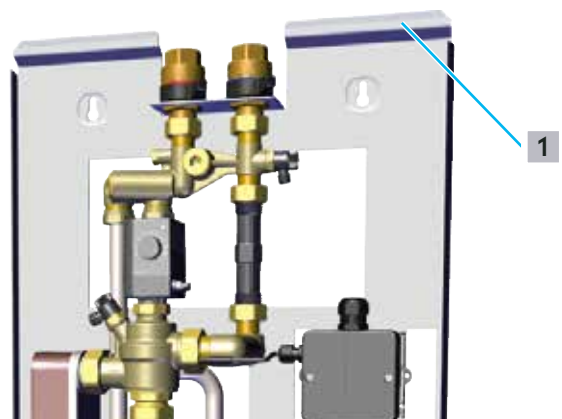
Abb. 19: Aufputzhaube montieren
