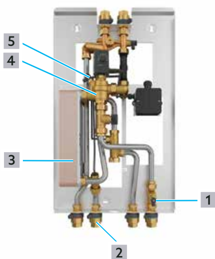
Abb. 21: Wärmeübertrager ausbauen und reinigen
