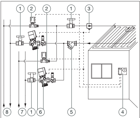
Abb. 7: Einbaubeispiel 2: Vierleitersystem
