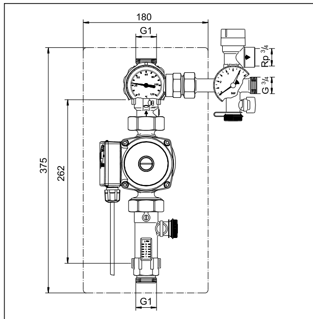
Coloana de pompare „Regusol 130“
