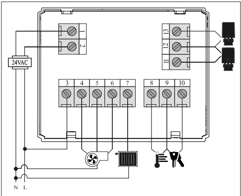
Abb. 6: Anschlussschema 1152065
