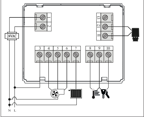
Abb. 5: Anschlussschema 1152064
