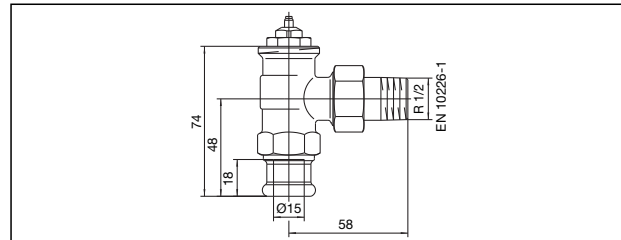
Maße Eckventil
