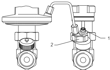
Abb. 6.1: „Hycoco DTZ“, Darstellung Impulsleitungsanschlusses, (Einbau im Rücklauf)
