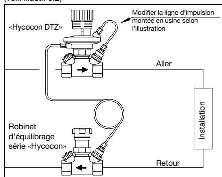
Illustr. 6.3: «Hycocn DTZ» Montage sur l'aller (seulement DN 32 + 40)
