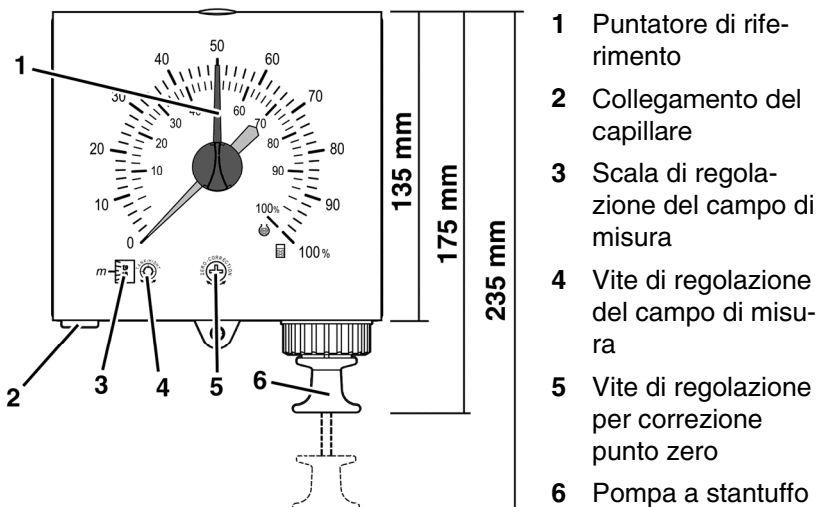
Fig.1 Vista frontale
