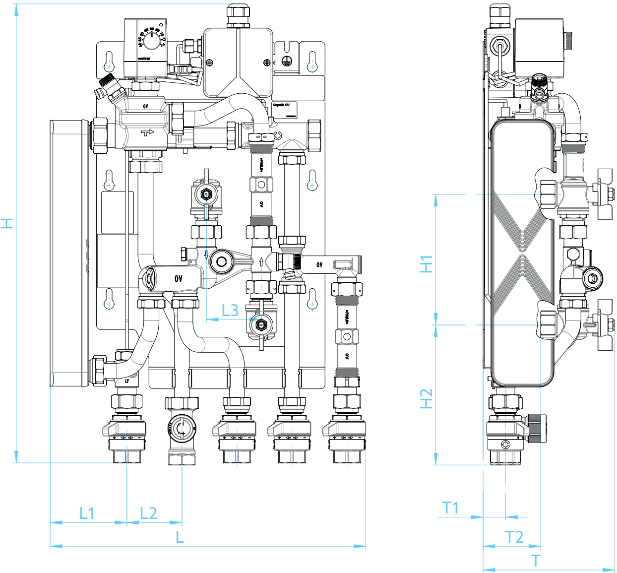
Fig. 6: Encombrements
