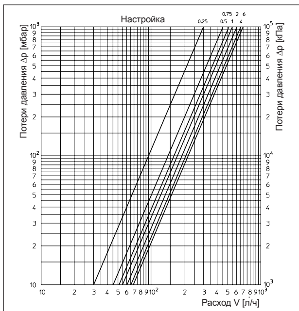
Регулирующ. вставка, 2К Р-отклон., преднастройка байпаса 1,4 (25%)
