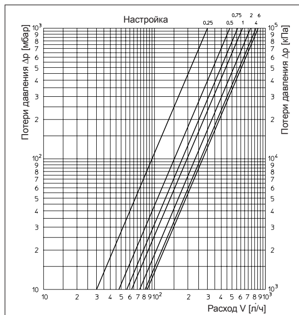
Регулирующ. вставка, 2К Р-отклон., преднастройка байпаса 1,9 (50%)
