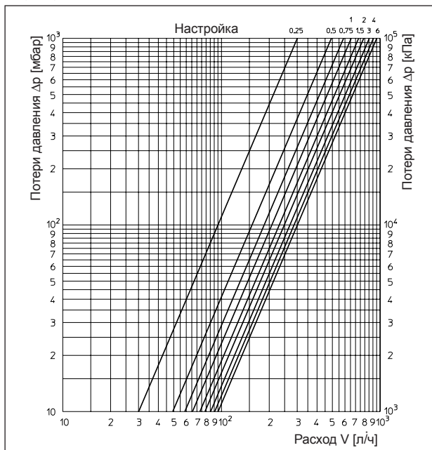
Регулирующ. вставка, 2К Р-отклон., преднастройка байпаса 2,3 (75%)
