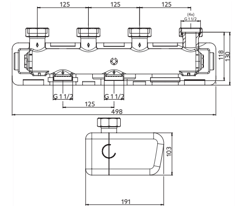
Abb. 2: Abmessungen
