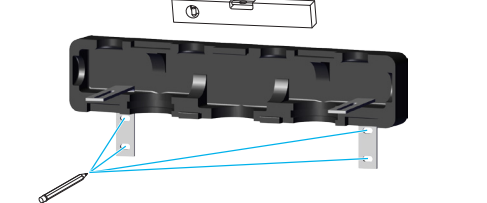
Abb. 5: Bohrlöcher markieren
