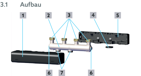
Abb. 1: Aufbau
