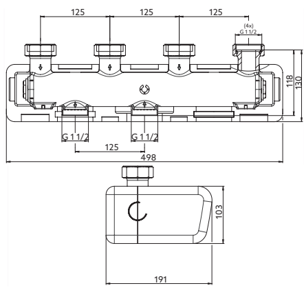
Fig. 2: Encombrements
