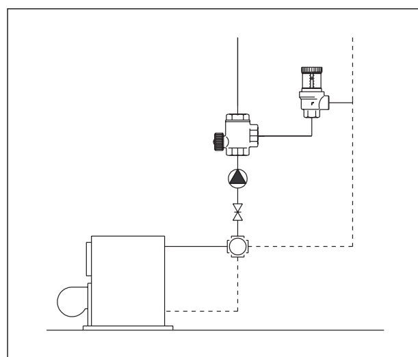
Schéma d'installation
