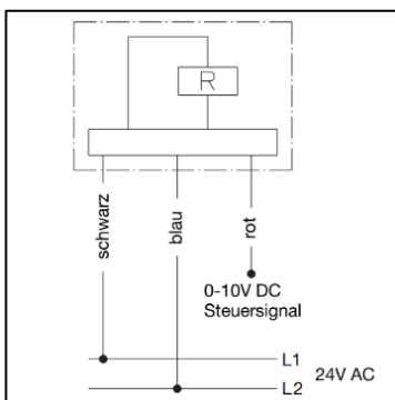
Schaltbild
