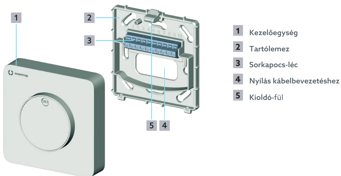
2: Beépítés F 90, F 100
