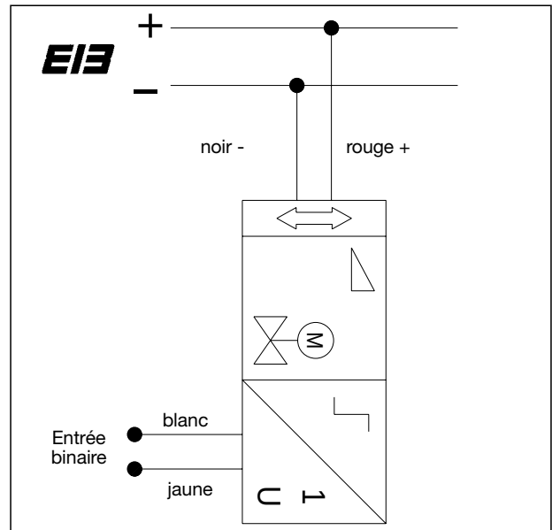
Schéma des connexions, réf. 115 60 65/75
