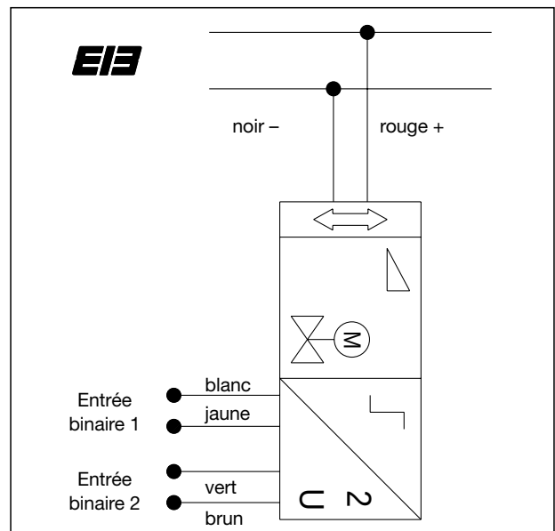
Schéma des connexions, réf. 115 60 66/76
