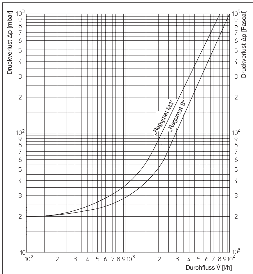
Durchflussdiagramm
