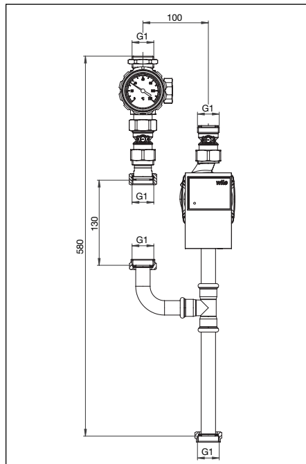
Fig. 4.3 Encombrements
