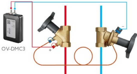
图 7： 连接图 OV-DMC3
