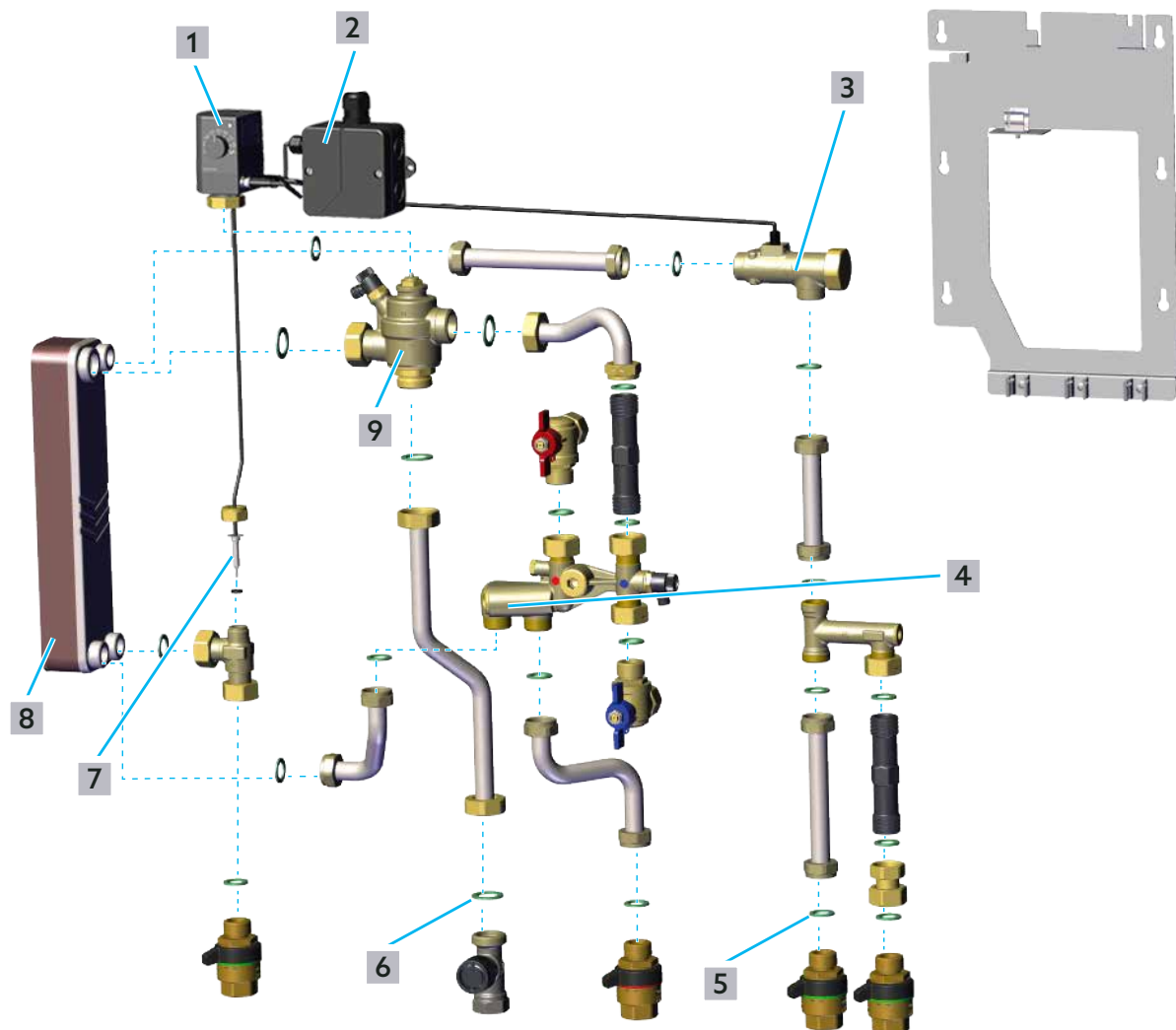
Abb. 8: Ersatzteile
