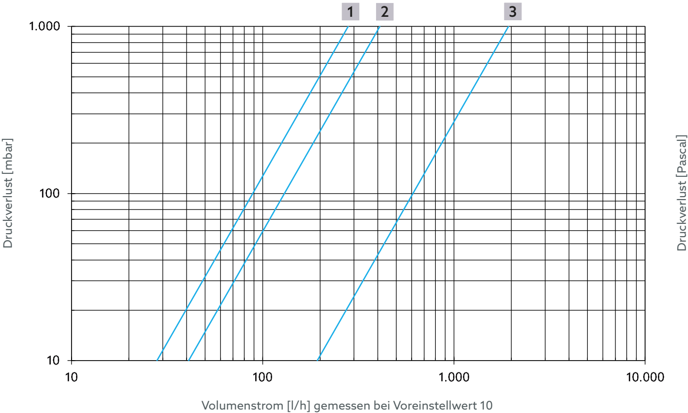
Abb. 19: Volumenstrom Thermische Regelung für Artikelnummer 4202506, 4202606, 4202706, 4202806
