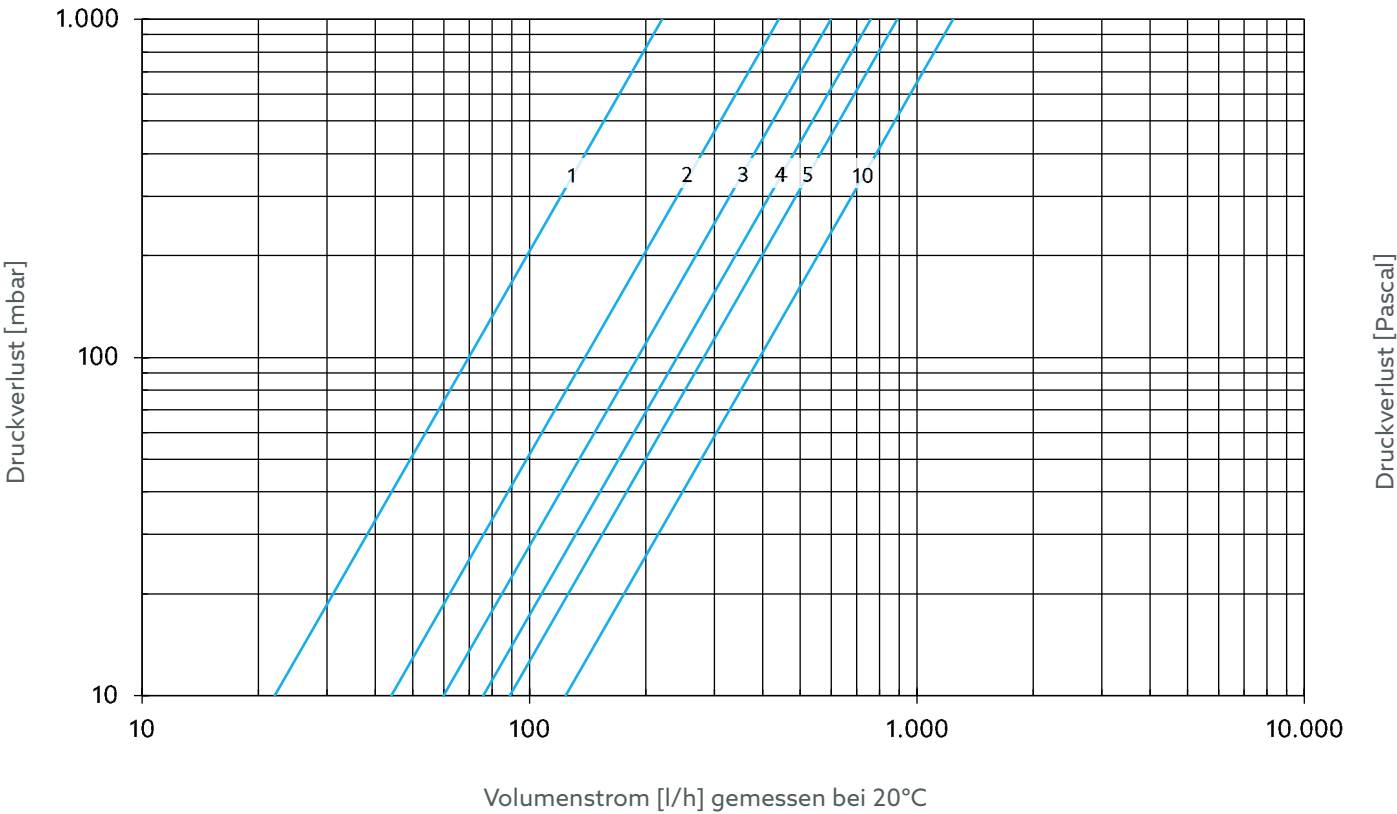
Abb. 15: Volumenstromvoreinstellung DN 15
