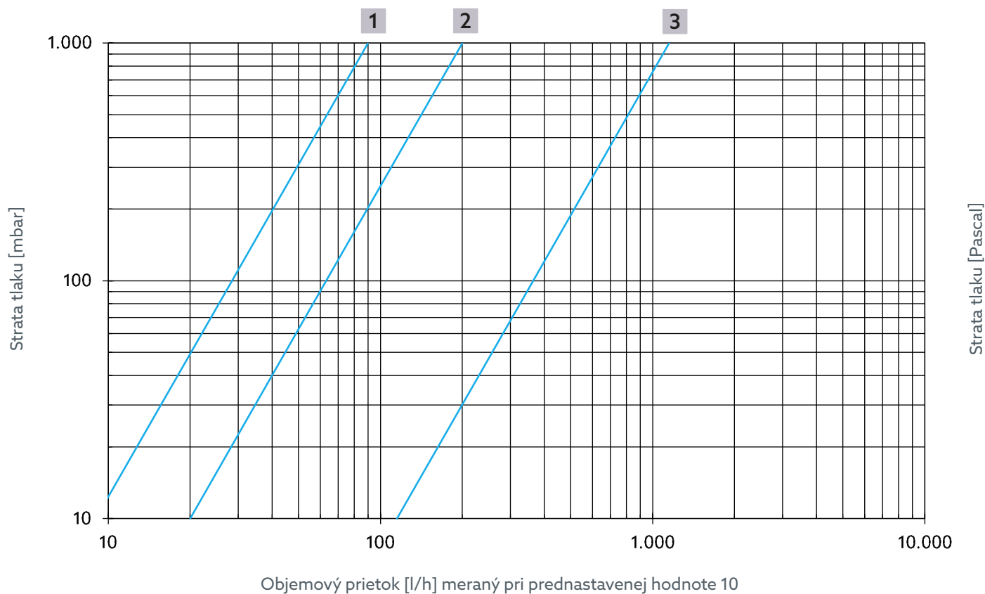
Obr. 17: Objemový prietok termoregulácie pre číslo položky 4202504, 4202604, 4202704, 4202804
