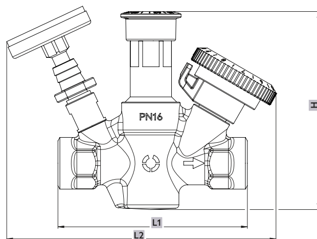
Obr. 2: Bočné rozmery
