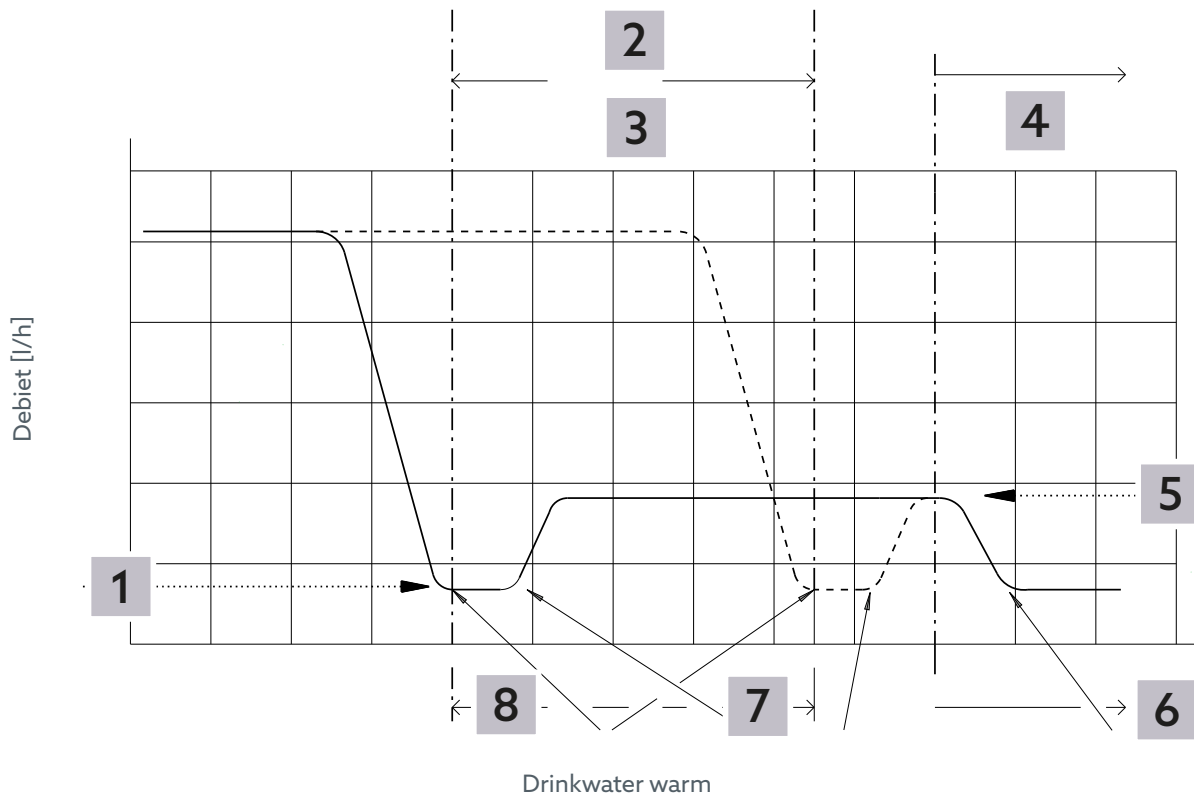
Afb. 6: Thermische regeling
