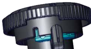
Obr. 14: Prednastavenie zablokovévané
