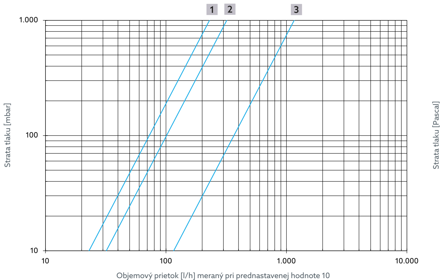
Obr. 18: Objemový prietok termoregulácie pre číslo položky 4202553 a 4202753
