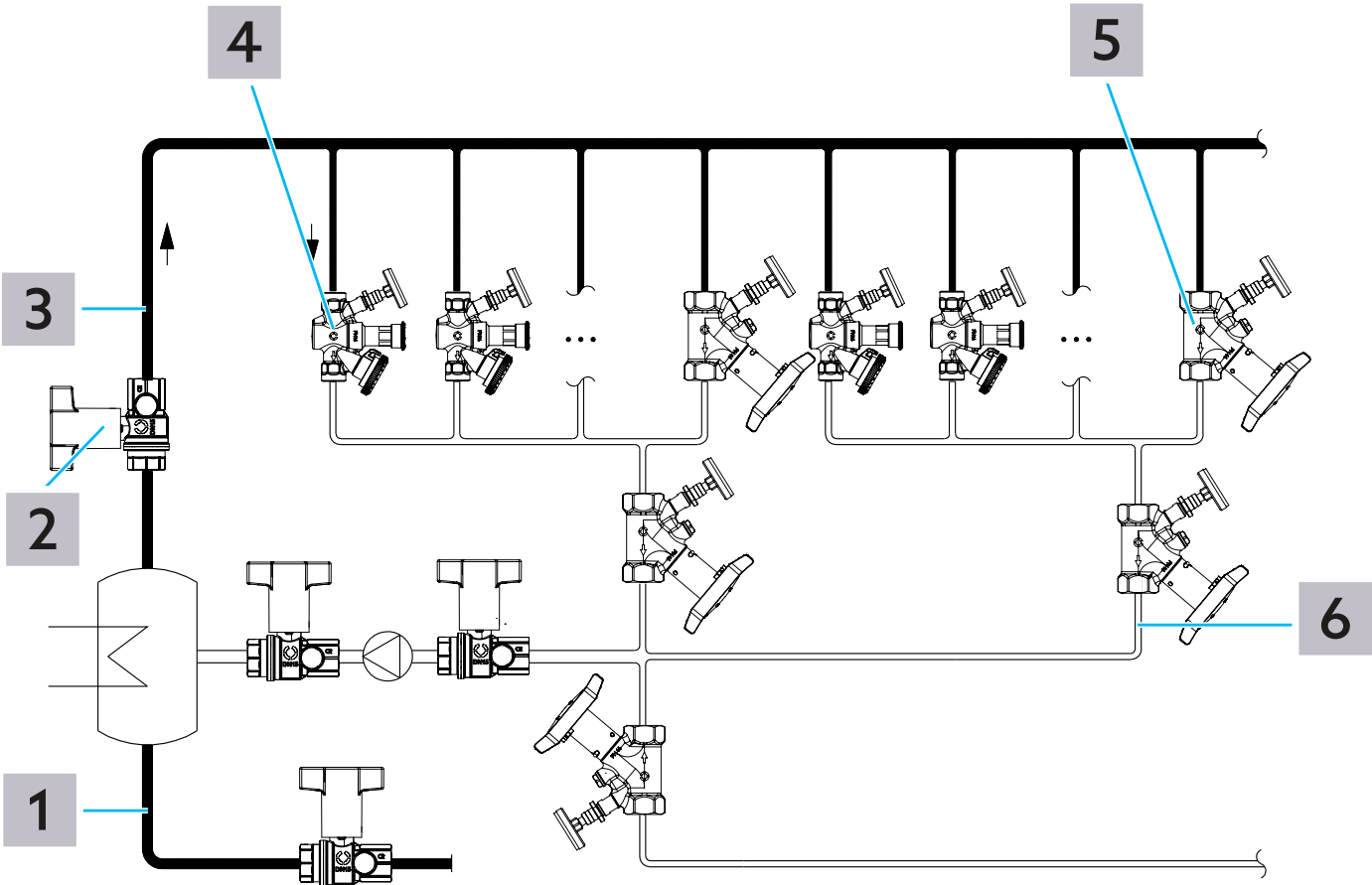
Рис. 4: Схема системы
