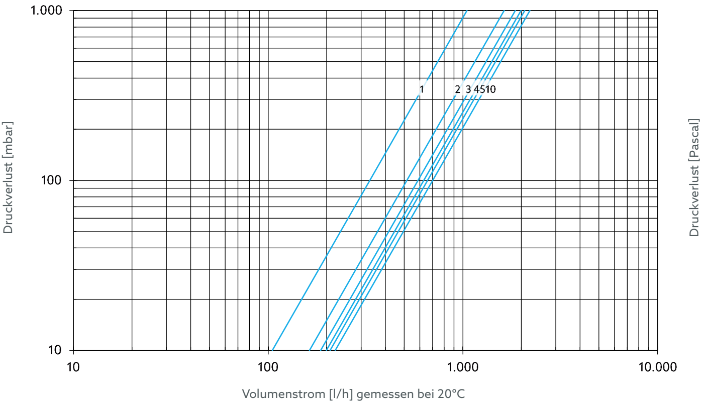
Abb. 16: Volumenstromvoreinstellung DN 20
