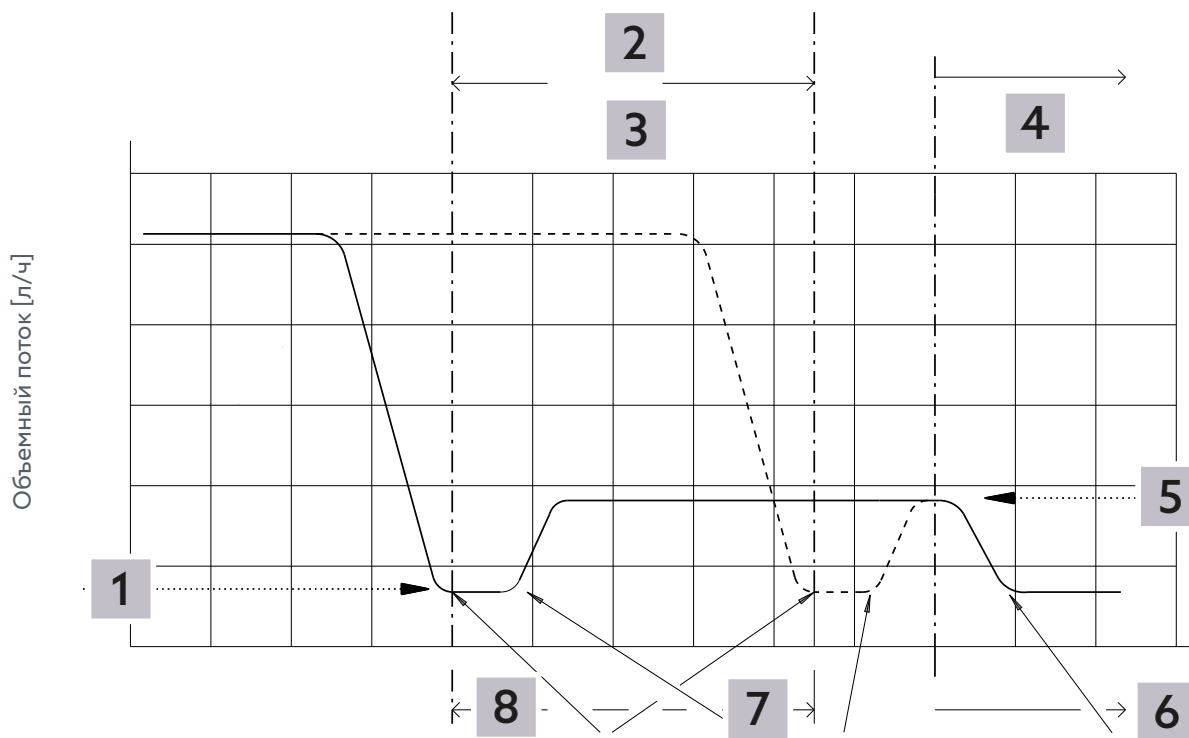
Рис. 6: Поведение при регулировке тепла
