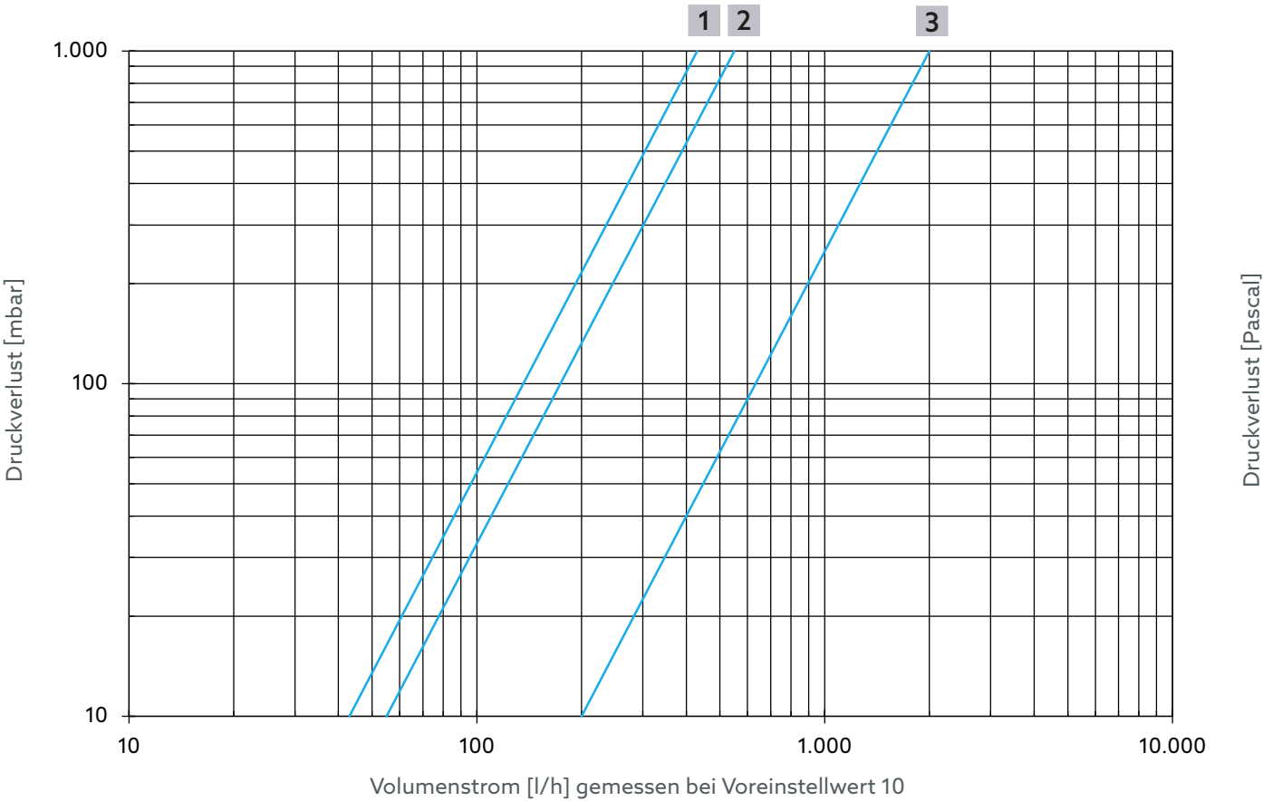
Abb. 20: Volumenstrom Thermische Regelung für Artikelnummer 4202554 und 4202754
