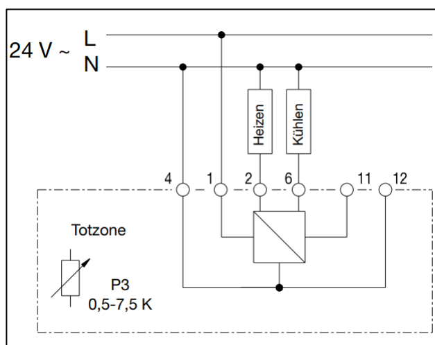
Schaltplan
