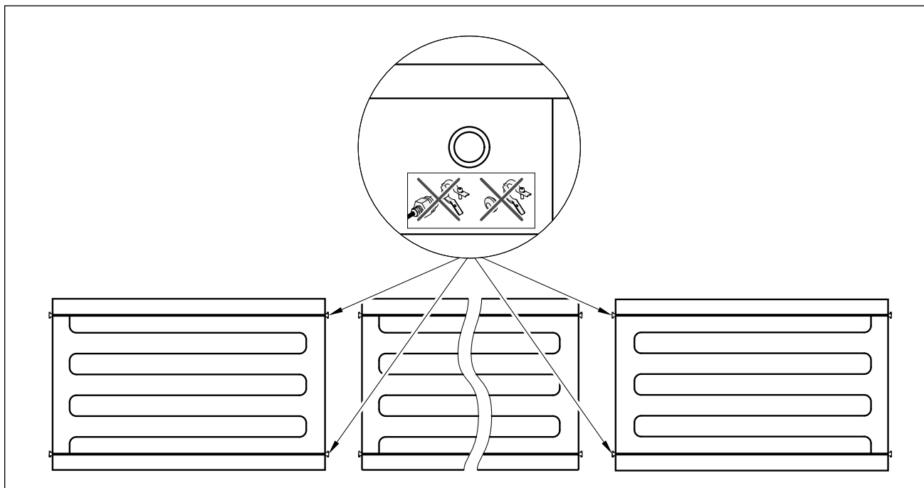
Abb. 15: Kollektoranordnung
